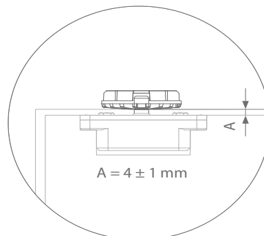
PLAFONDBEVESTIGING / MONTAGE AU PLAFOND / CEILING MOUNT / DECKENMONTAGE
