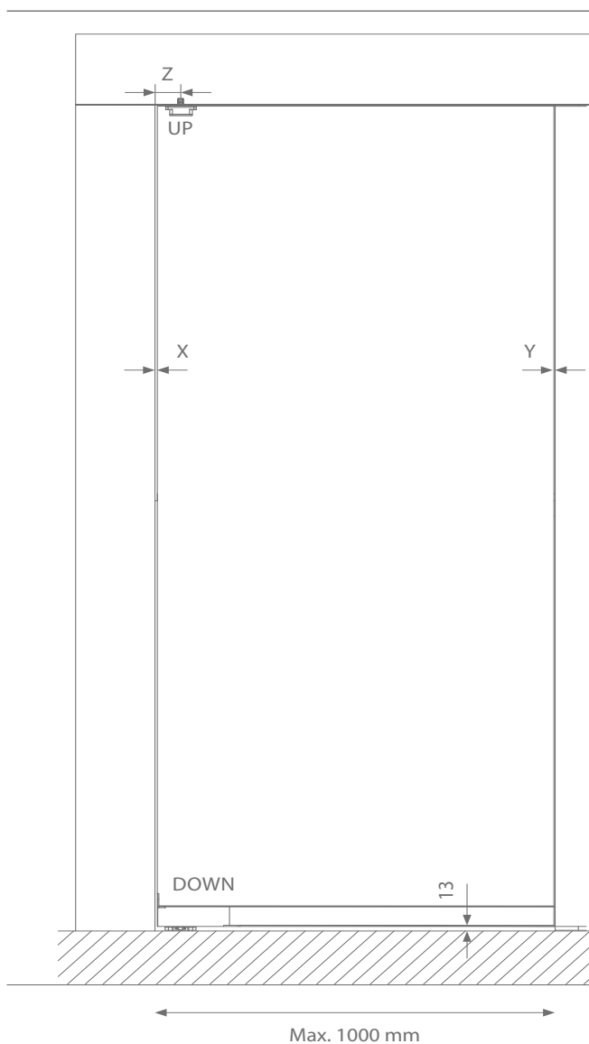
PLAFONDBEVESTIGING / MONTAGE AU PLAFOND / CEILING MOUNT / DECKENMONTAGE
