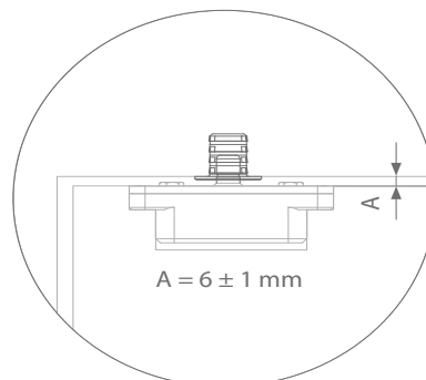
LINTEEL MONTAGE / MONTAGE SOUS LINTEAU / LINTEL MOUNT / MONTAGE IM STURZ /
