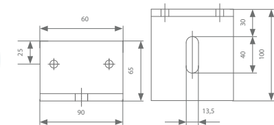
Draagstuk 131.910
