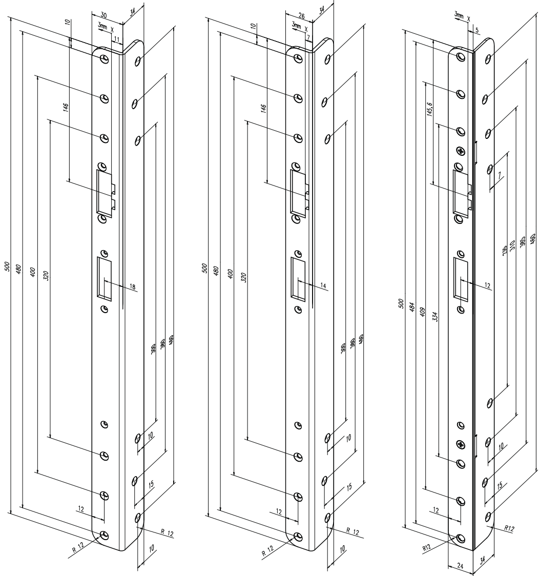
Renovierungswinkelschließbleche
