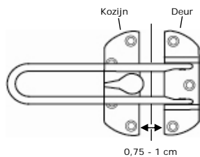
Situatie B - rechte haak
