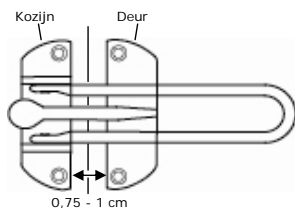
Situatie A - kromme haak
